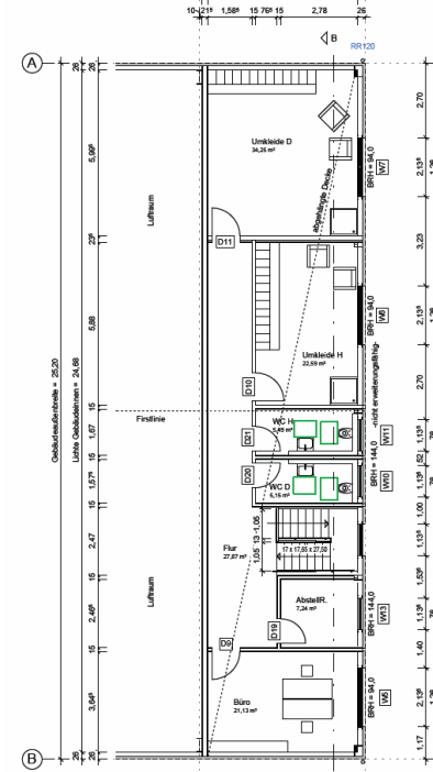
OG (Räume)
